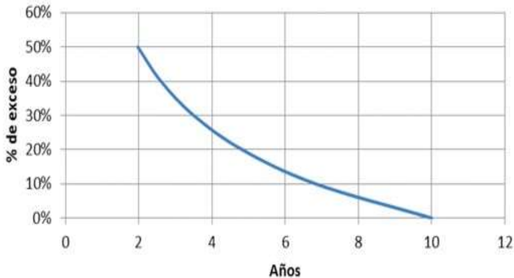
GRÁFICO 2: Duración del pavimento según el exceso de cargas.
